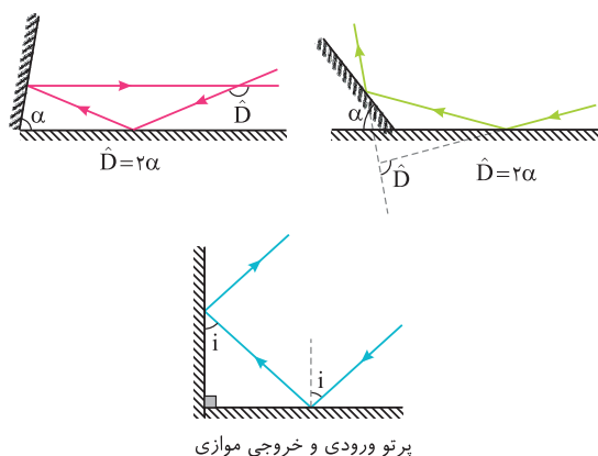
پرتو ورودی و خروجی موازی
