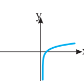
اکیداً صعودی، y = \log_a x, a > 1
