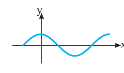
غیریکنوا، y = \cos x
