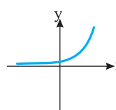
اکیداً صعودی، y = a^x, a > 1
