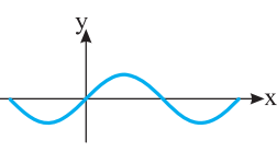
غیریکنوا، y = \sin x
