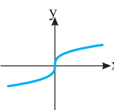
اکیداً صعودی، y = \sqrt[3]{x}
