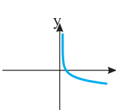
اکیداً نزولی، y = \log_a x, 0 < a < 1
