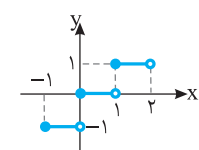
صعودی، y = [x]
