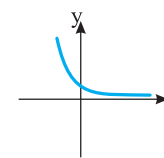
اکیداً نزولی، y = a^x, 0 < a < 1
